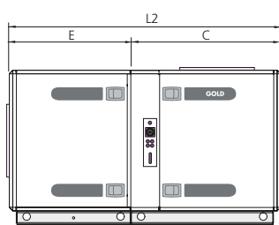
Ventilateur + filtre
