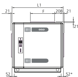
Ventilateur
