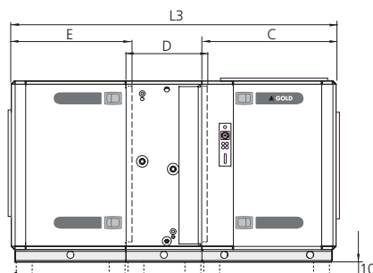
Ventilateur + filtre + échangeur de chaleur à batterie
