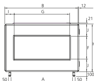
Ventilateur
