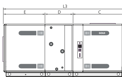
Ventilateur + filtre + échangeur de chaleur à batterie
