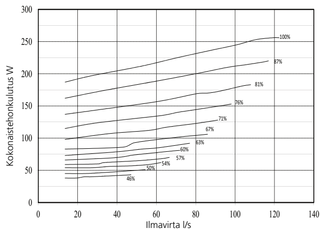
Tehonkulutus
